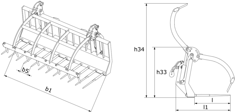
Widły do obornika z chwytakiem - widło krokodyl - Rysunek wymiarowy
