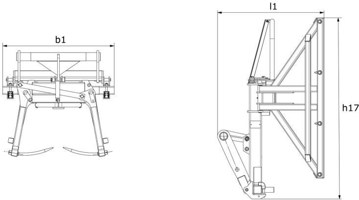
Захват для тюков -Intensive- - габаритный чертеж
