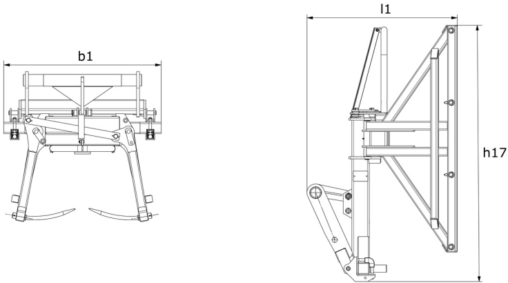
Захват для тюков -Intensive- - габаритный чертеж
