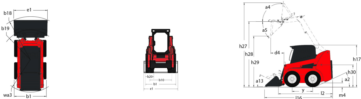
1350R NXT2 - габаритный чертеж
