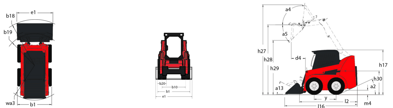
1640R (iT4) - Diagrama dimensional
