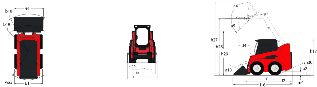
1640R (iT4) - габаритный чертеж
