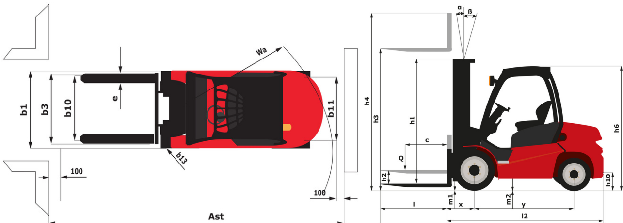
MI 40 G FOB - габаритный чертеж
