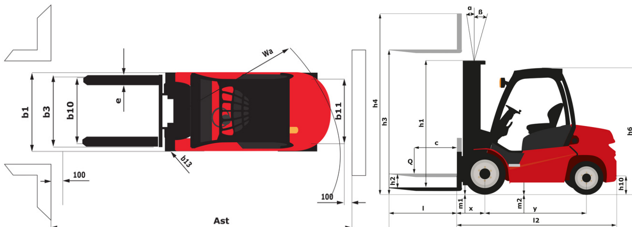
MI 40 G FOB - габаритный чертёж
