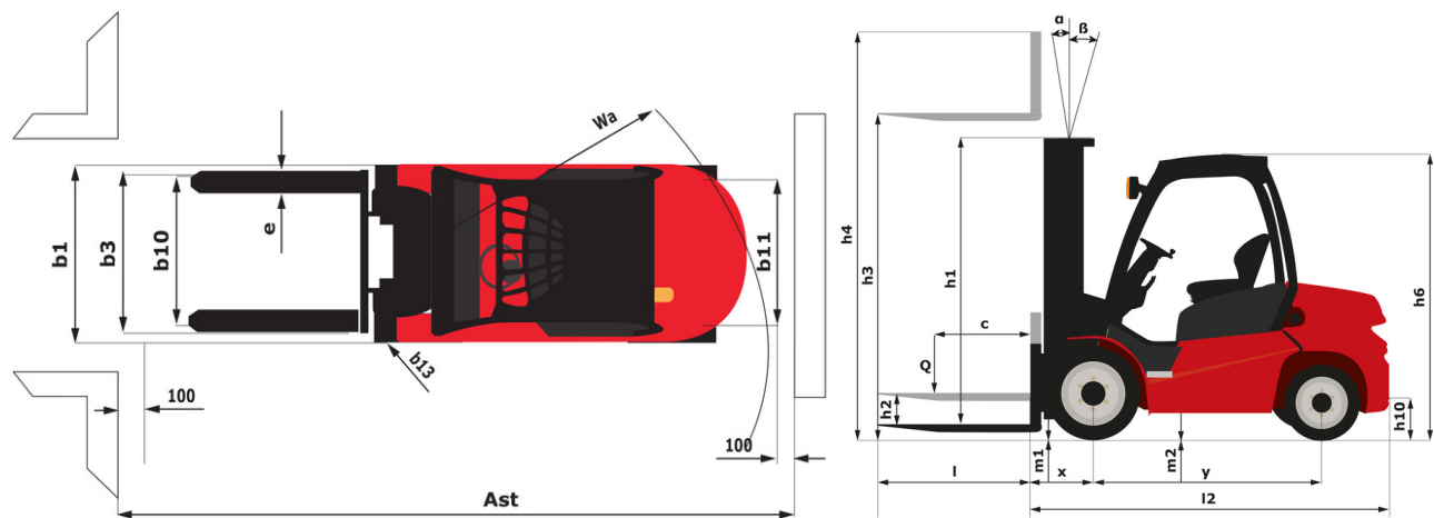
MI 45 G FOB - габаритный чертеж
