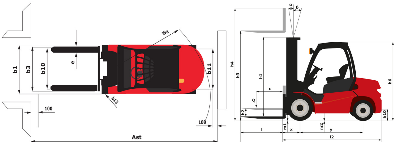
MI 50 G FOB - габаритный чертёж
