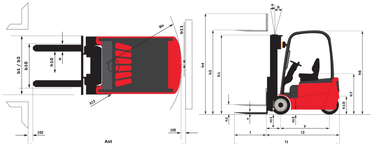
ME 315 C FOB - габаритный чертеж
