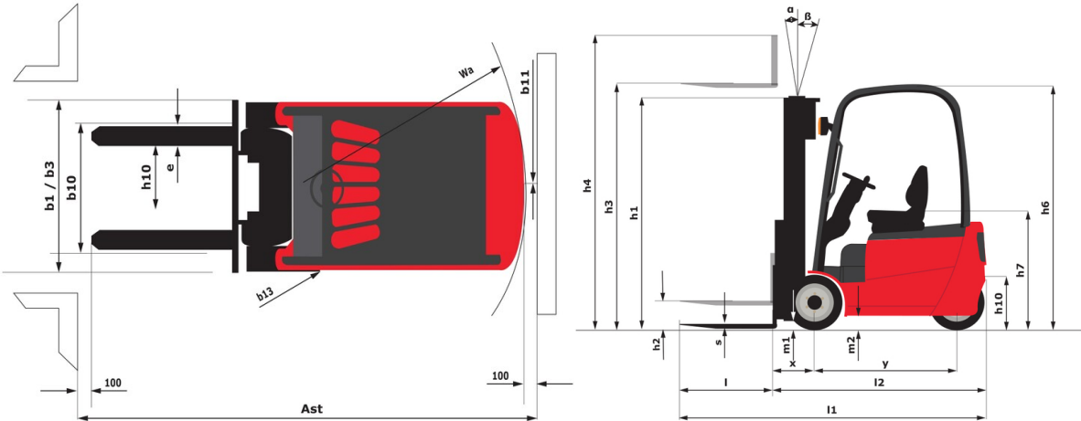
ME 316 FOB - габаритный чертеж
