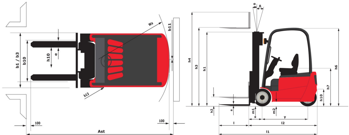
ME 425C FOB - габаритный чертеж
