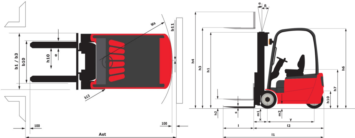
ME 425 FOB - габаритный чертеж
