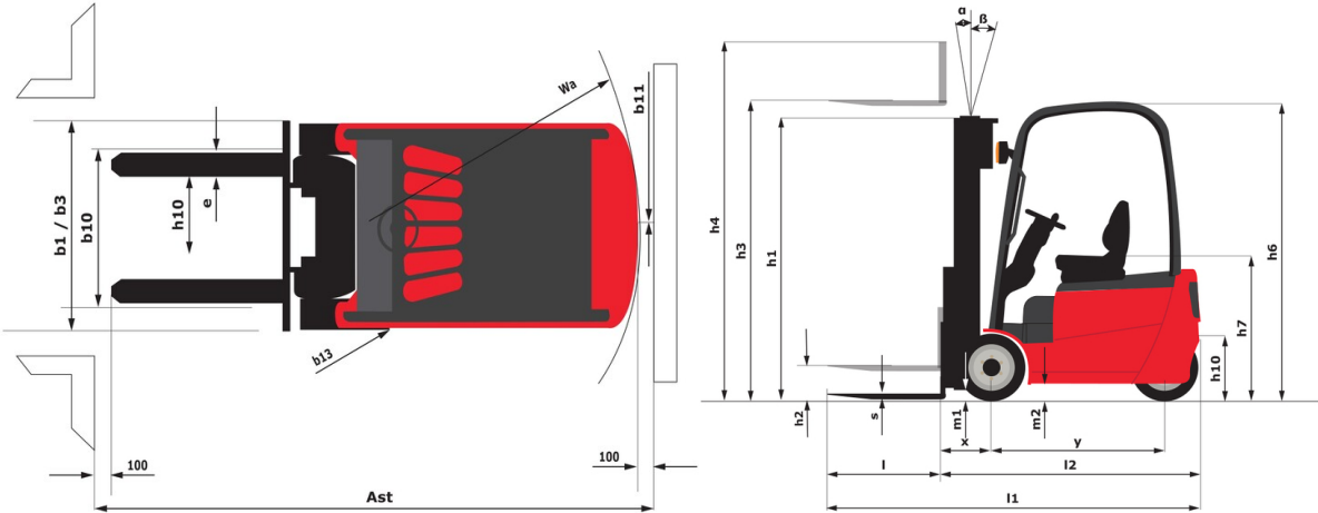
ME 430 FOB - Diagrama dimensional
