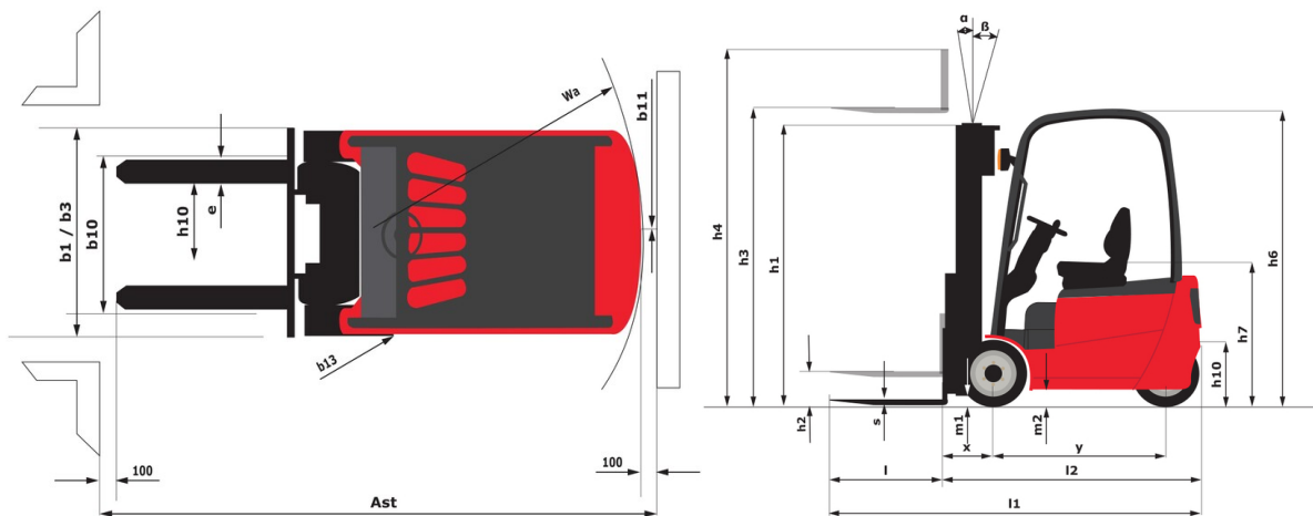
ME 430 FOB - Diagrama dimensional
