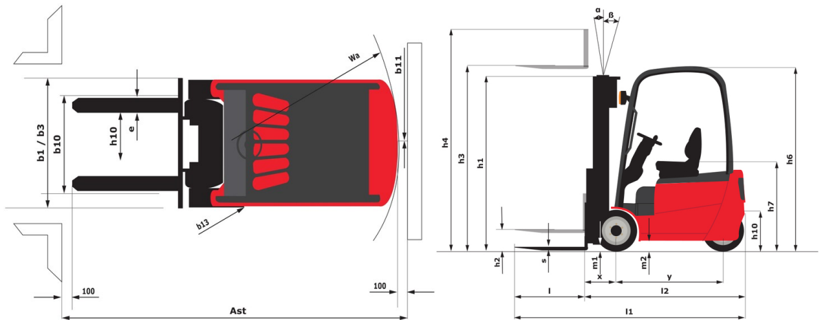
ME 445 FOB - Diagrama dimensional
