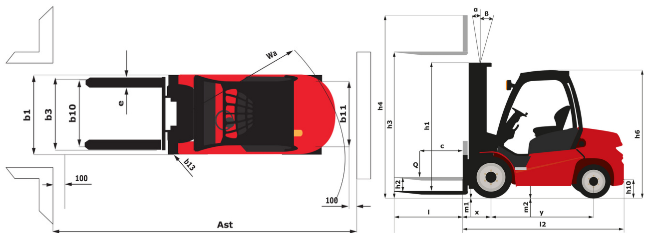
MI 60 G FOB - габаритный чертеж
