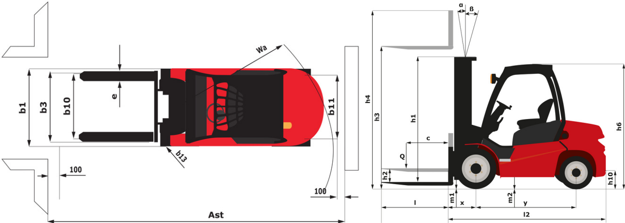
MI 70 G FOB - габаритный чертеж
