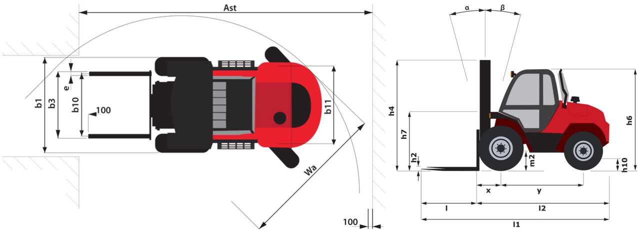
M 50-4 D ST5 - Maßzeichnung
