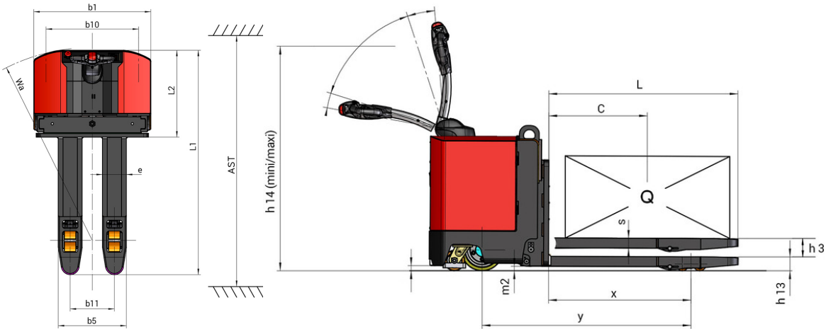
EP 740 - Maßzeichnung
