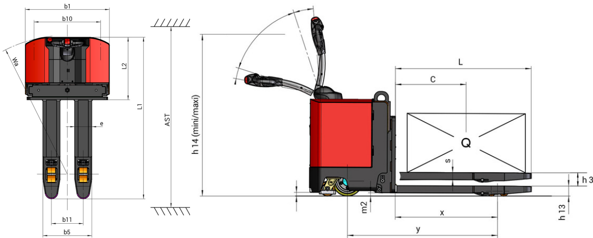
EP 750 - Maßzeichnung
