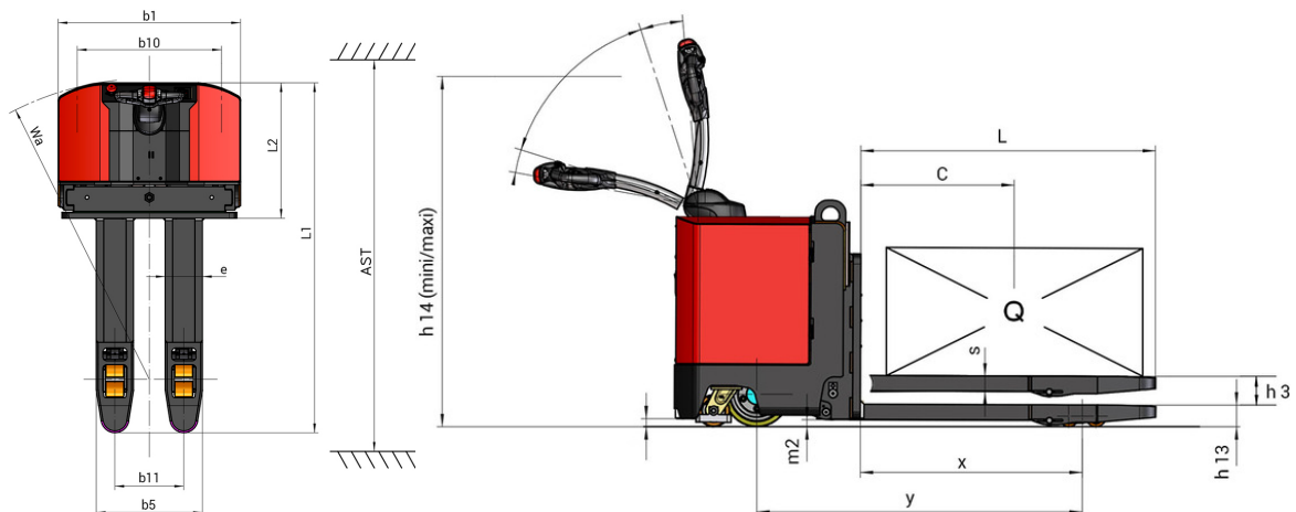
EP 750 - Tekening met afmetingen
