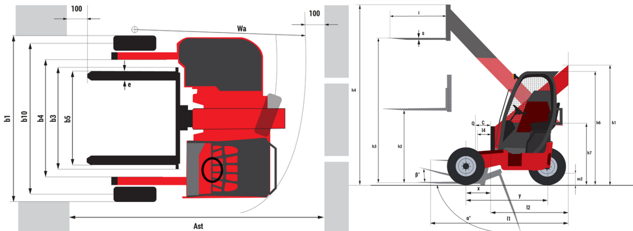
TMT 27S Y ST5 - 寸法図
