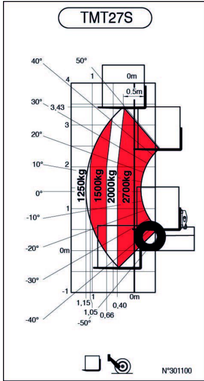
スタビライザー未使用時フォーク-メートル法
