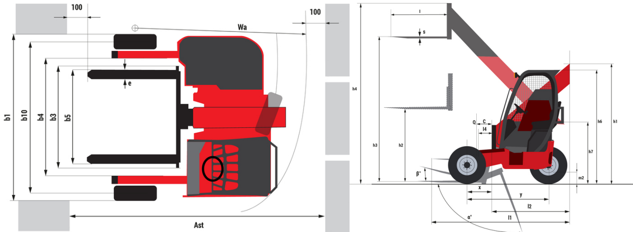
TMT 25I Y ST5 - Diagrama dimensional
