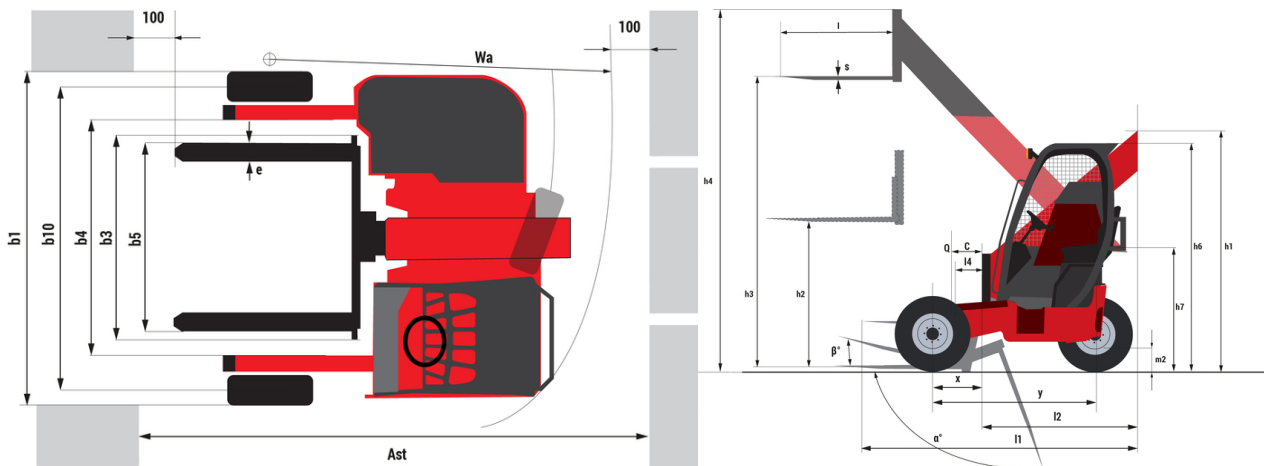
TMT 25I Y ST5 - Tekening met afmetingen
