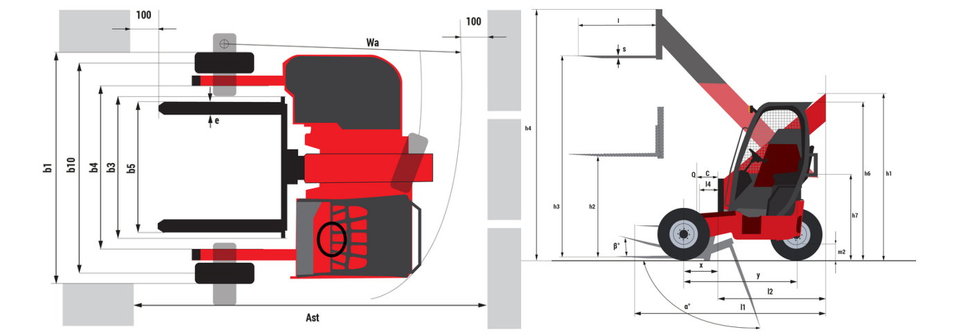
TMT 55 HT 4W Y ST5 - Schémas d'encombrement
