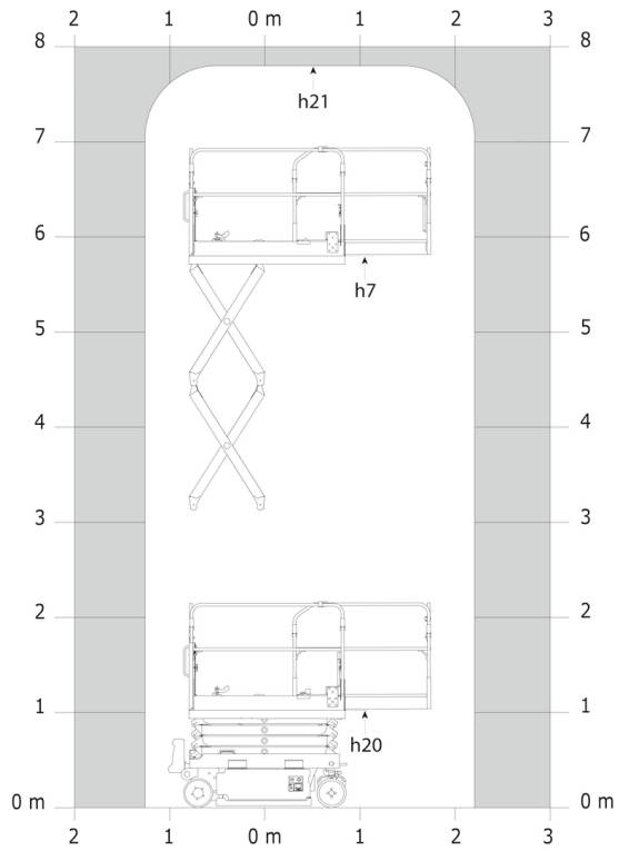
Diagramma di carico per piattaforme portapersona
