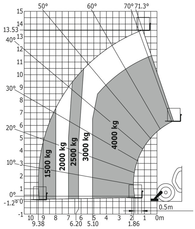
Maszyna na stabilizatorach, z obrotową wieżą, z widłami
