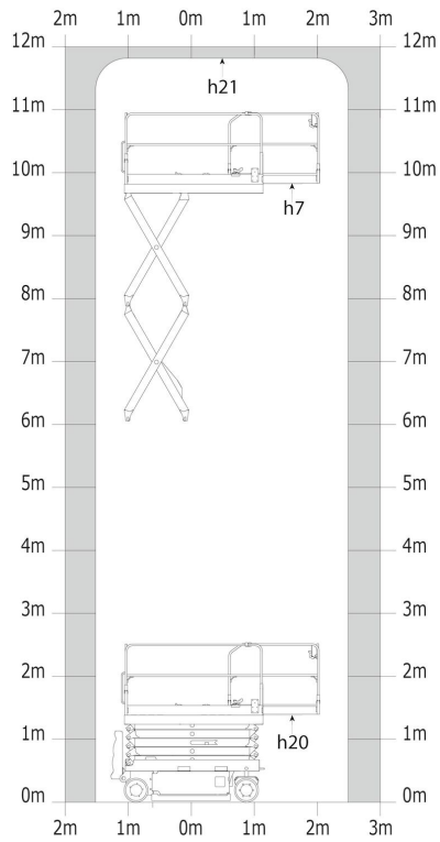
Gráfico da carga para plataforma elevatória (métrico)
