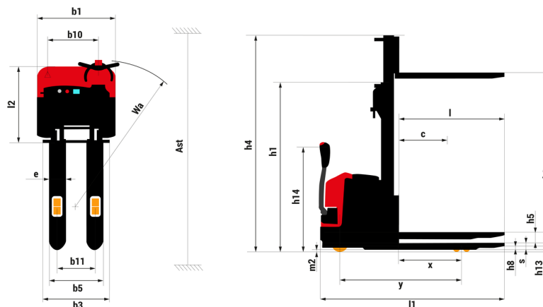
ES 316 L Easy - Tekening met afmetingen
