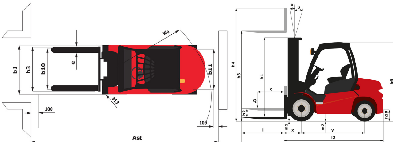
MI 20 D ST5 FOB - Diagrama dimensional
