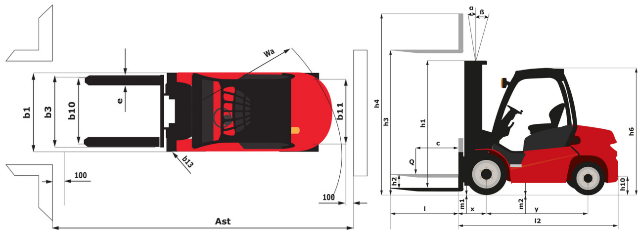
MI 15 G ST5 FOB - Diagrama dimensional
