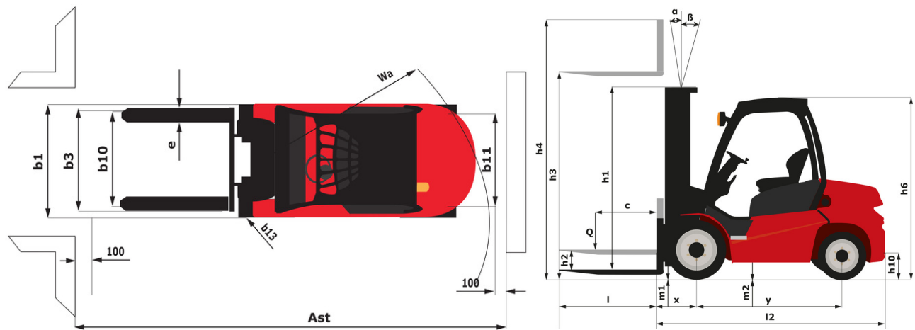
MI 15 G ST5 FOB - габаритный чертеж
