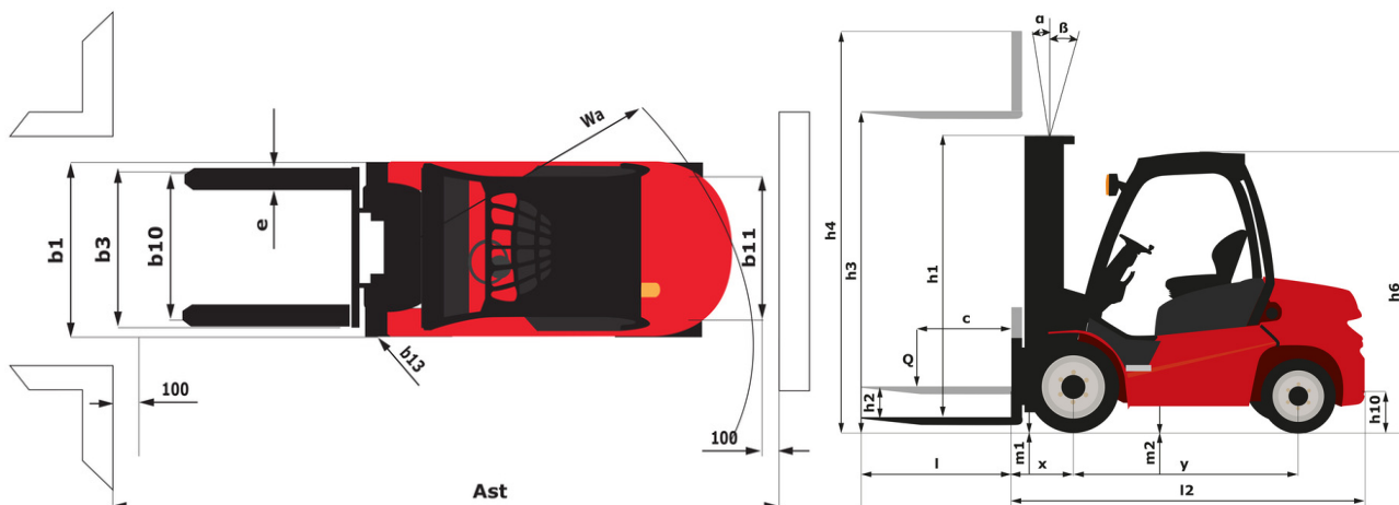
MI 20 G ST5 FOB - габаритный чертеж
