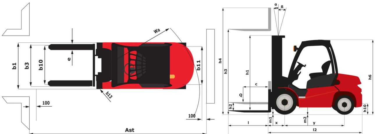
MI 80 D ST5 - Rysunek wymiarowy
