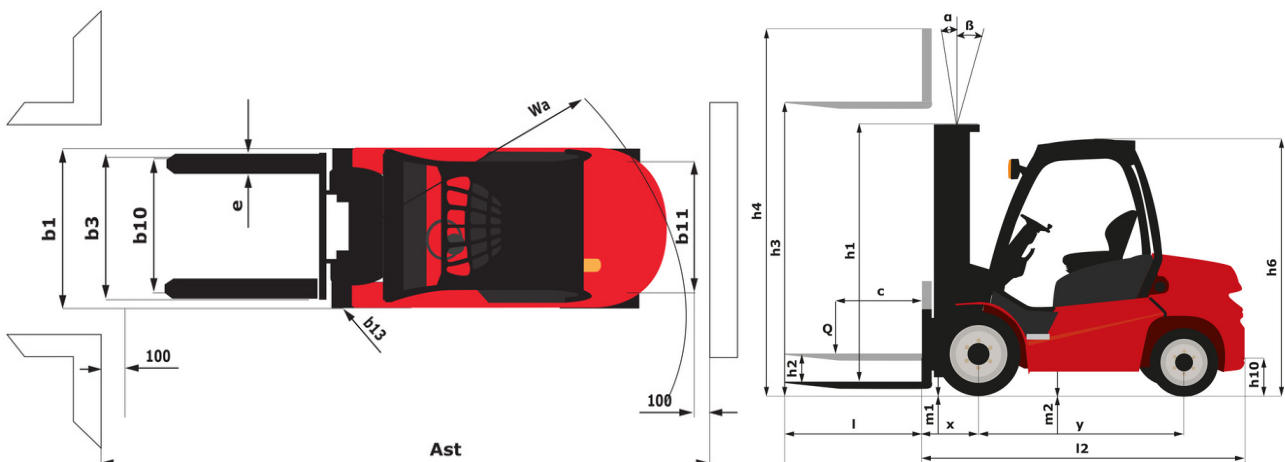
MI 100 D ST5 - Rysunek wymiarowy
