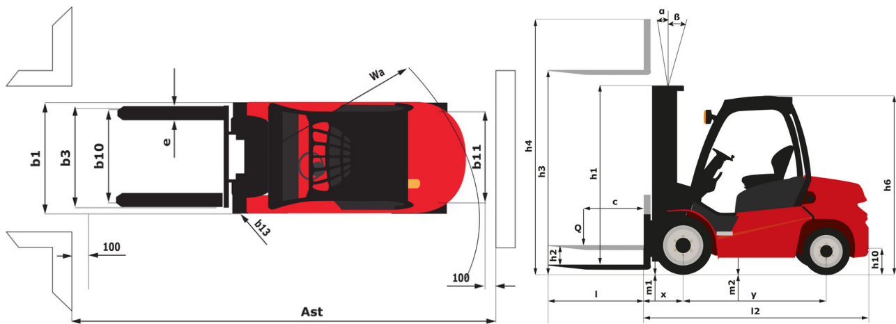
MI-X 40 D FOB - Schémas d'encombrement
