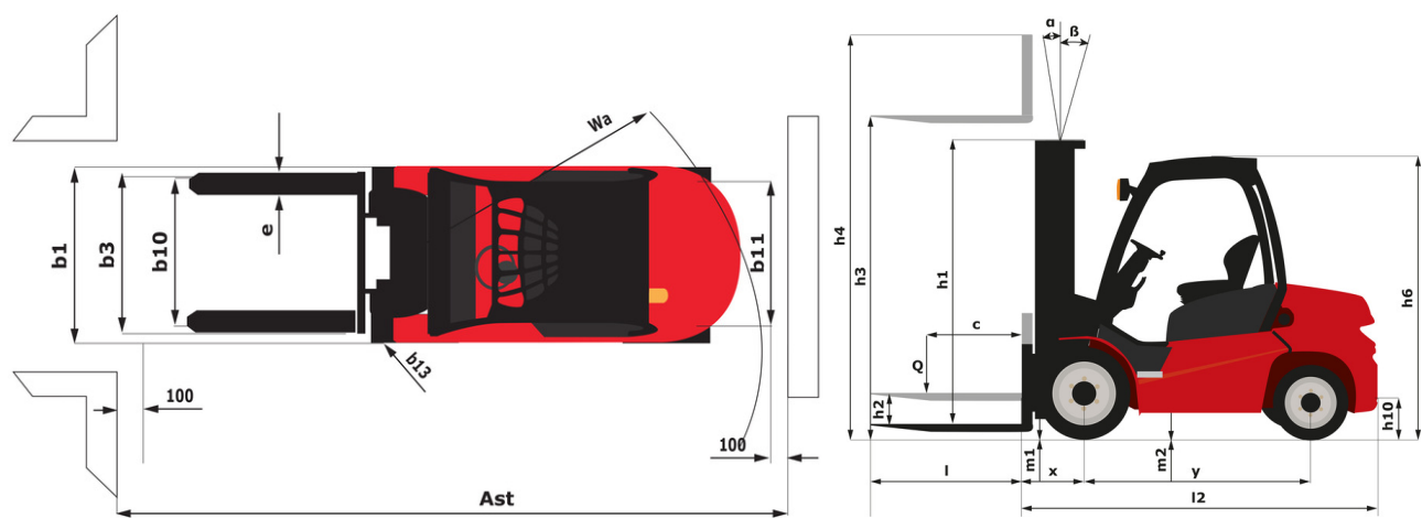
MI-X 40 D FOB - Schémas d'encombrement
