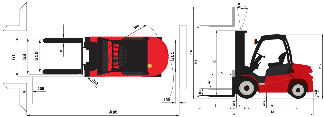
MI-X 55 D - габаритный чертеж
