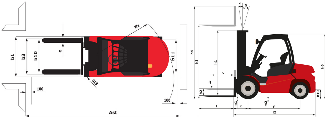
MI 40 G ST5 - Disegno quotato
