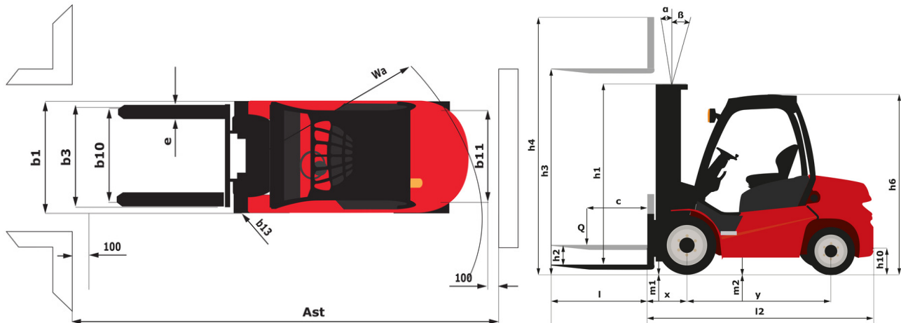
MI 45 G ST5 - Diagrama dimensional
