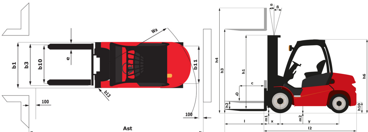
MI 55 G ST5 - Tekening met afmetingen
