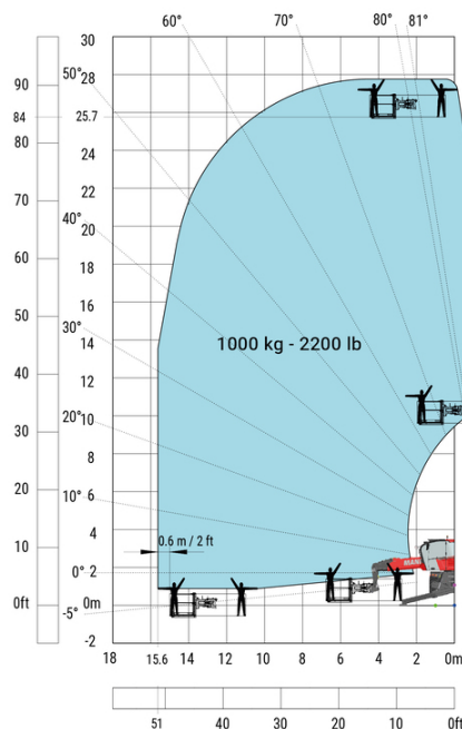
Rotación sobre estabilizadores bajados, con plataforma de 1.000 kg
