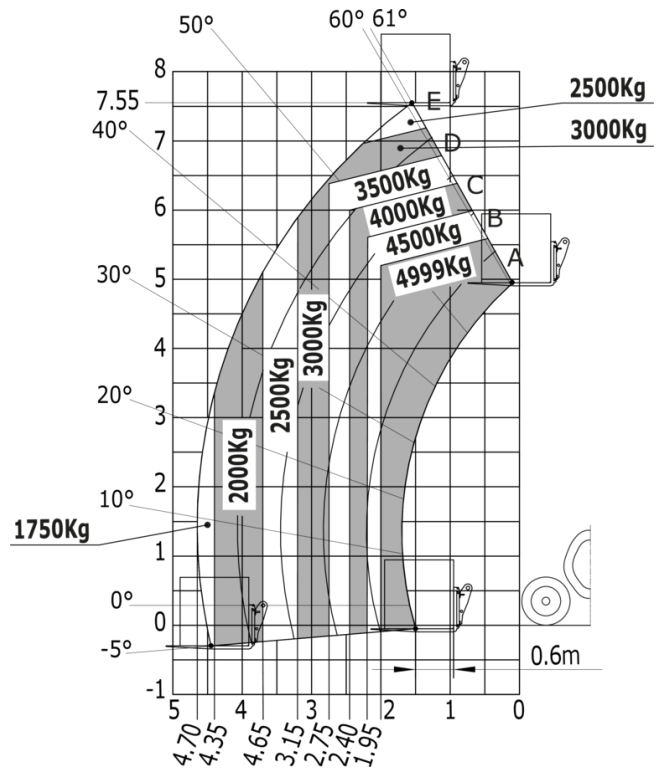
スタビライザ未使用時LC600mmフォーク-メートル法
