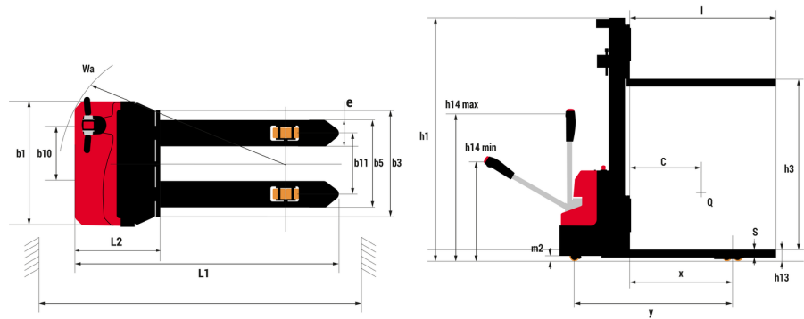
ES 112 Easy - габаритный чертеж
