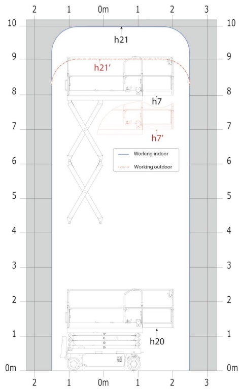
作業範囲図 メートル法
