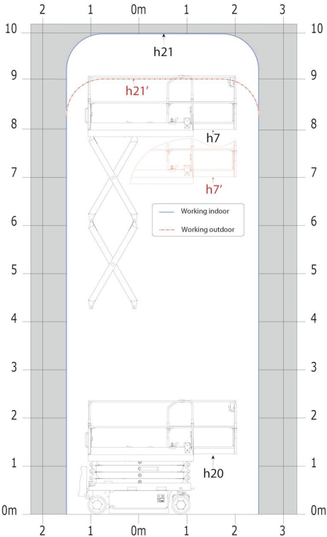
Gráfico da carga para plataforma elevatória (métrico)
