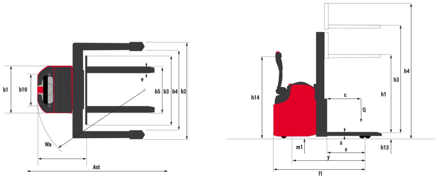
ES 720 4W - Diagrama dimensional
