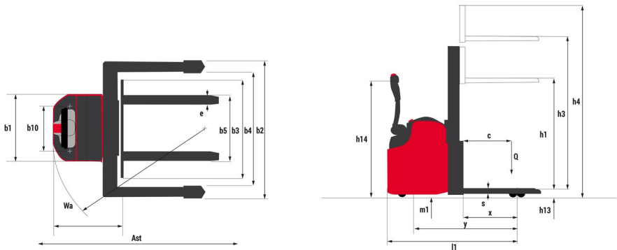
ES 412 LE - Diagrama dimensional
